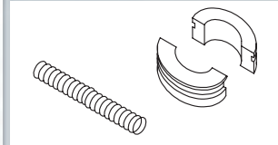
3-Backenkupplung mit Feder 3-Shoe clutch with spring
