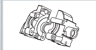
Getriebegehäuse vorne/hinten Gear housing front/rear
