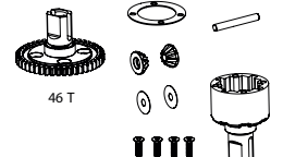
Mitteldiff komplett Centerdiff complete
