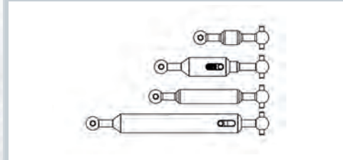
1:14 Antriebswellen-Set (4) 6x6 Längenausgleich +/-5mm 1:14 Propeller shaft Set (4) 6x6 Length adjustment +/-5mm
